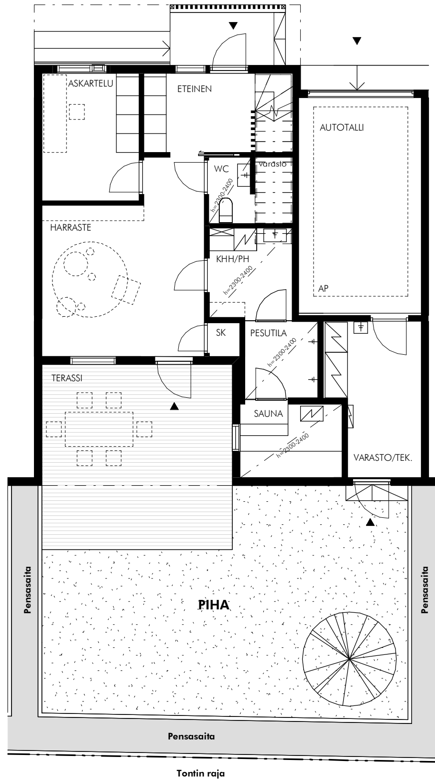
1. KERROS 1 : 100
