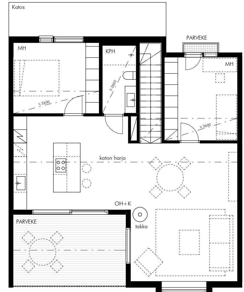
2. KERROS 1 : 100
